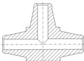
三通对焊接头 T-cock butt joint
