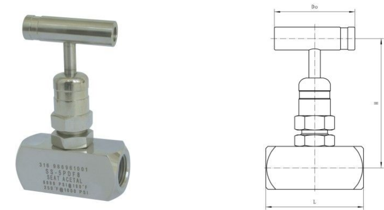
▲主要连接尺寸 General Dimensions
