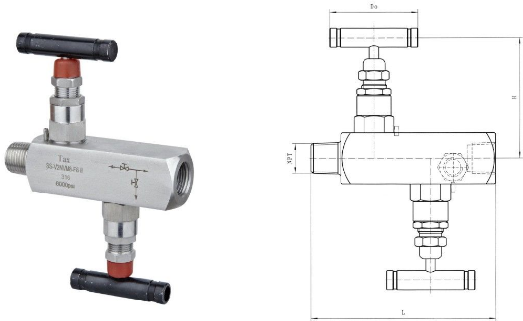
示意图 Schematic Diagram
